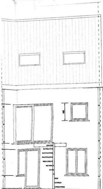
achtergevel
