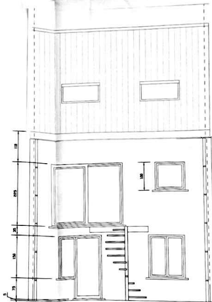
achtergevel
